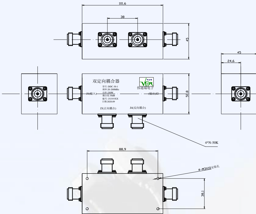
DDC-30-1外形及尺寸
