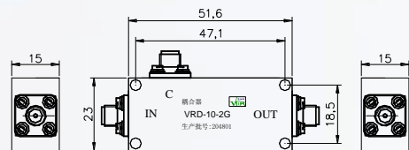
VRD-10-2G外形及尺寸
