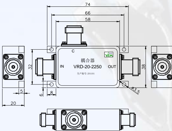
VRD-20-2250外形及尺寸
